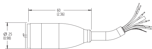
投入式电缆
