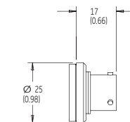
卡口插座MIL-C-26482
