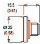
M12×15 5针
